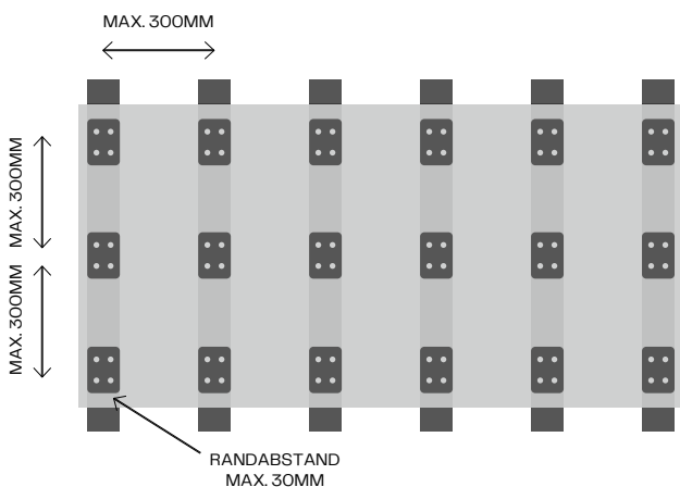
ABSTÄNDE DER VAKUUMSAUGER
