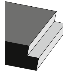
FALZAUSFRÄSUNG/TYP M Bild 36
