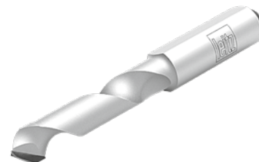
LEITZ-BOHRER SCHAFT 10 MM Bild 52
