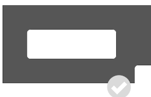
AUSFRÄSUNGEN IN DER MAX COMPACT PLATTE
