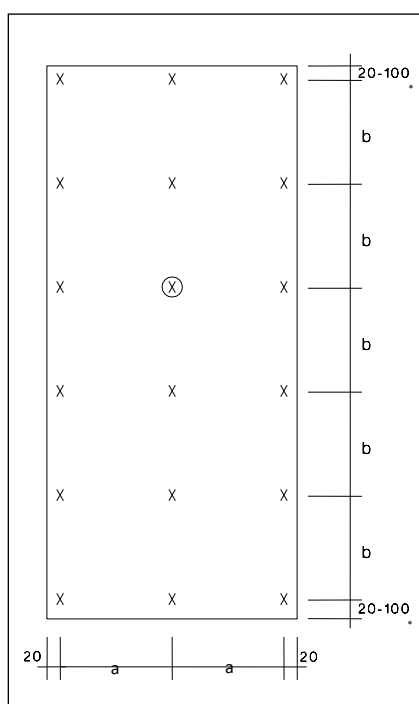
Figuur 2: 3 steunpunten per plaat
