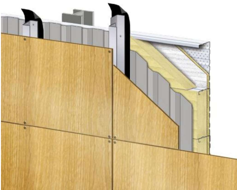
Figure 1 – Schéma de principe panneaux avec pare-pluie métallique
