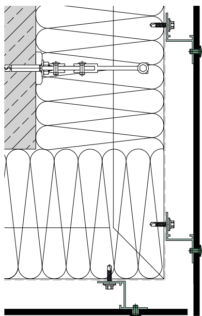
Außenecke A105
