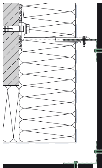
Außenecke A105
