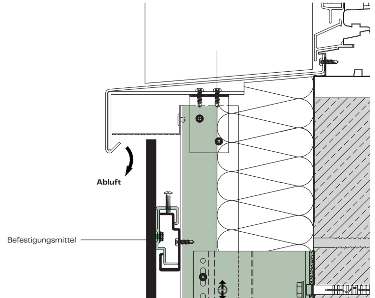
Fensterbankanschluss A102
