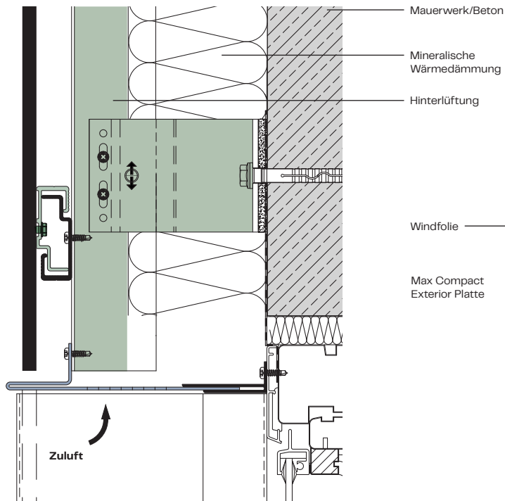
Fenstersturz A101
