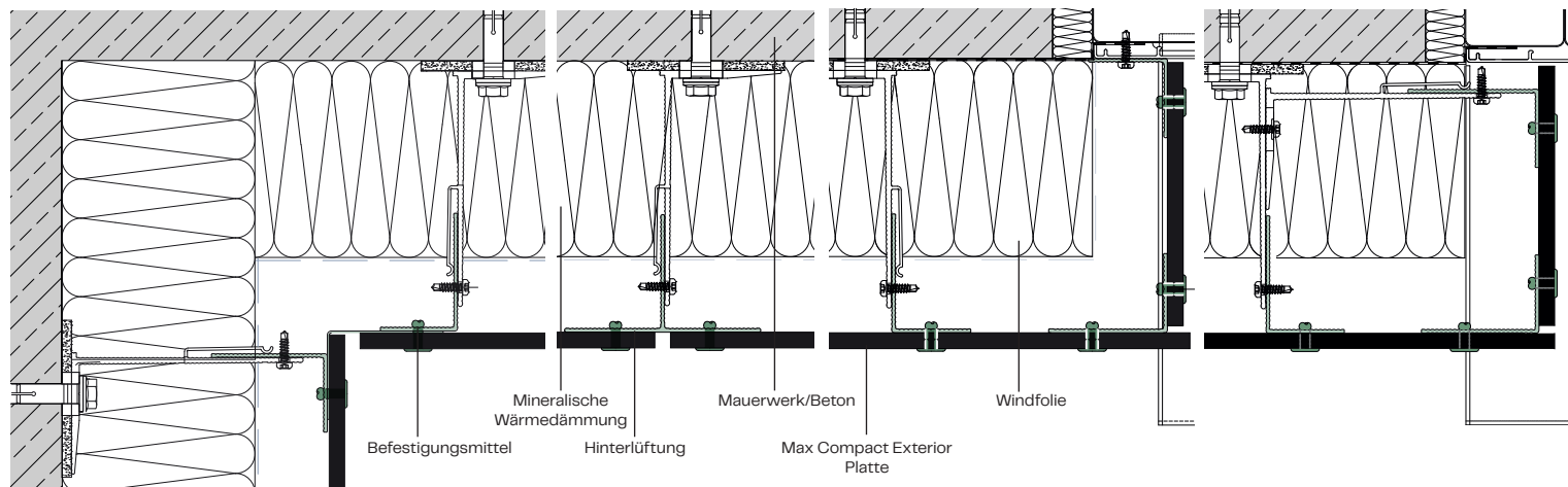
Innenecke A106
