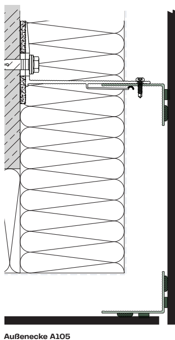
Außenecke A105
