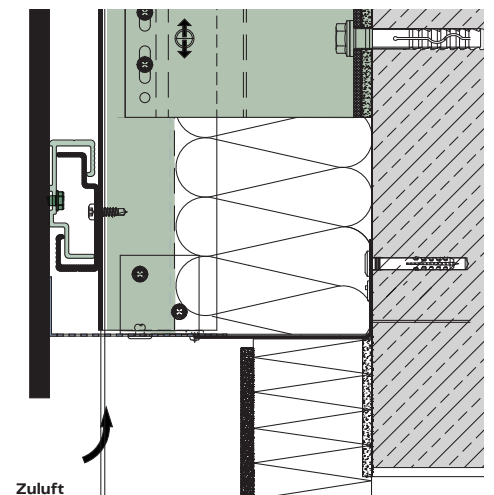
Sockelanschluss A103
